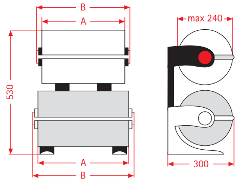
Aufsatz-Abroller dispenser attachement dérouleur superposable
